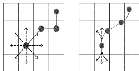
(a) A* 算法搜索路径 (b) Hybrid A* 算法搜索路径
