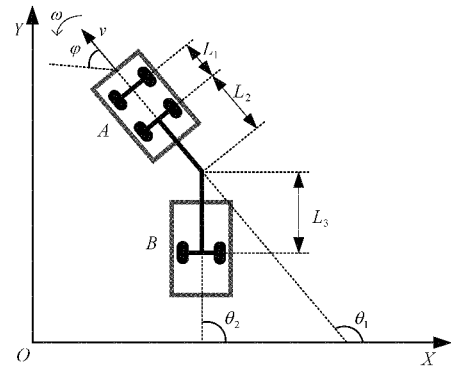
图 1 带一节拖挂车的移动机器人系统的数学模型
