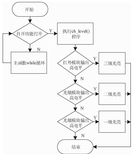
图 8 调级功能算法流程
