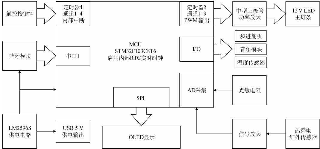
图 1 硬件系统方案
