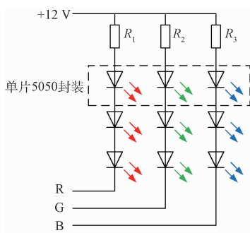
图 3 5 cm 长度灯条等效电路
