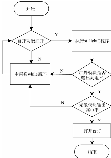
图 7 自开功能算法流程
