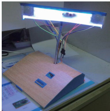
图 10 多功能智能台灯实物
