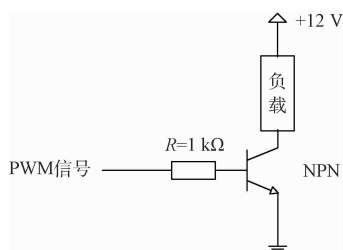
图 4 功率放大电路
